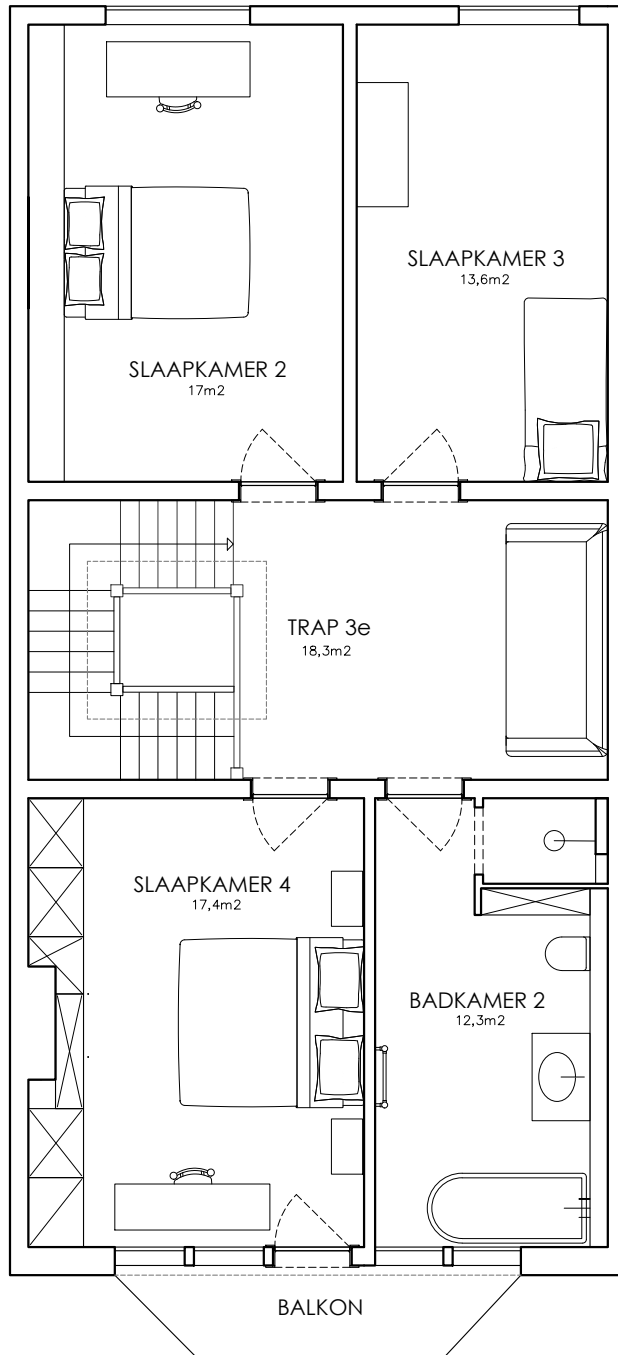
3e VERDIEPING
